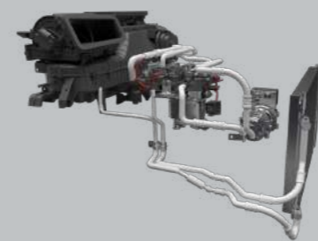
高効率ヒートポンプシステム： -30℃～60℃の広い温度範囲で稼働可能 高電圧システムの廃熱を吸収
