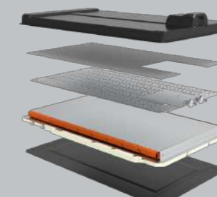
バッテリーパック： 直冷直熱メカニズムにより熱効率を20%向上 冬場の走行可能距離が10%アップ
